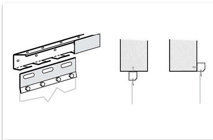
Dettagli dell'aggancio e del fissaggio interno/esterno vano.
